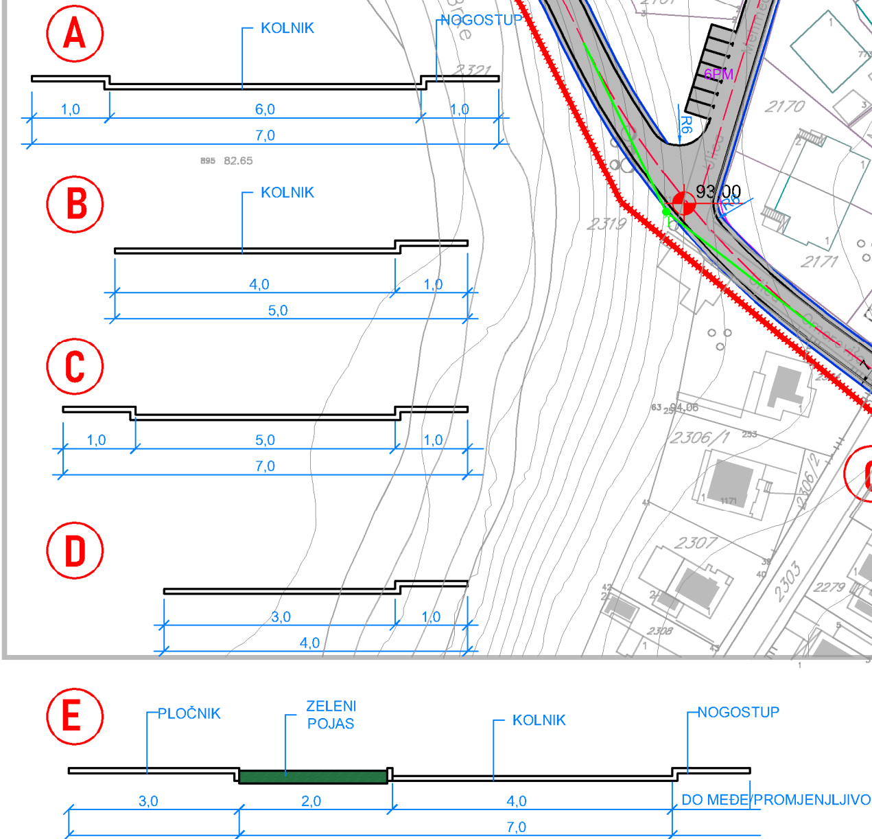
PROFILI SAOBRAĆAJNICA
